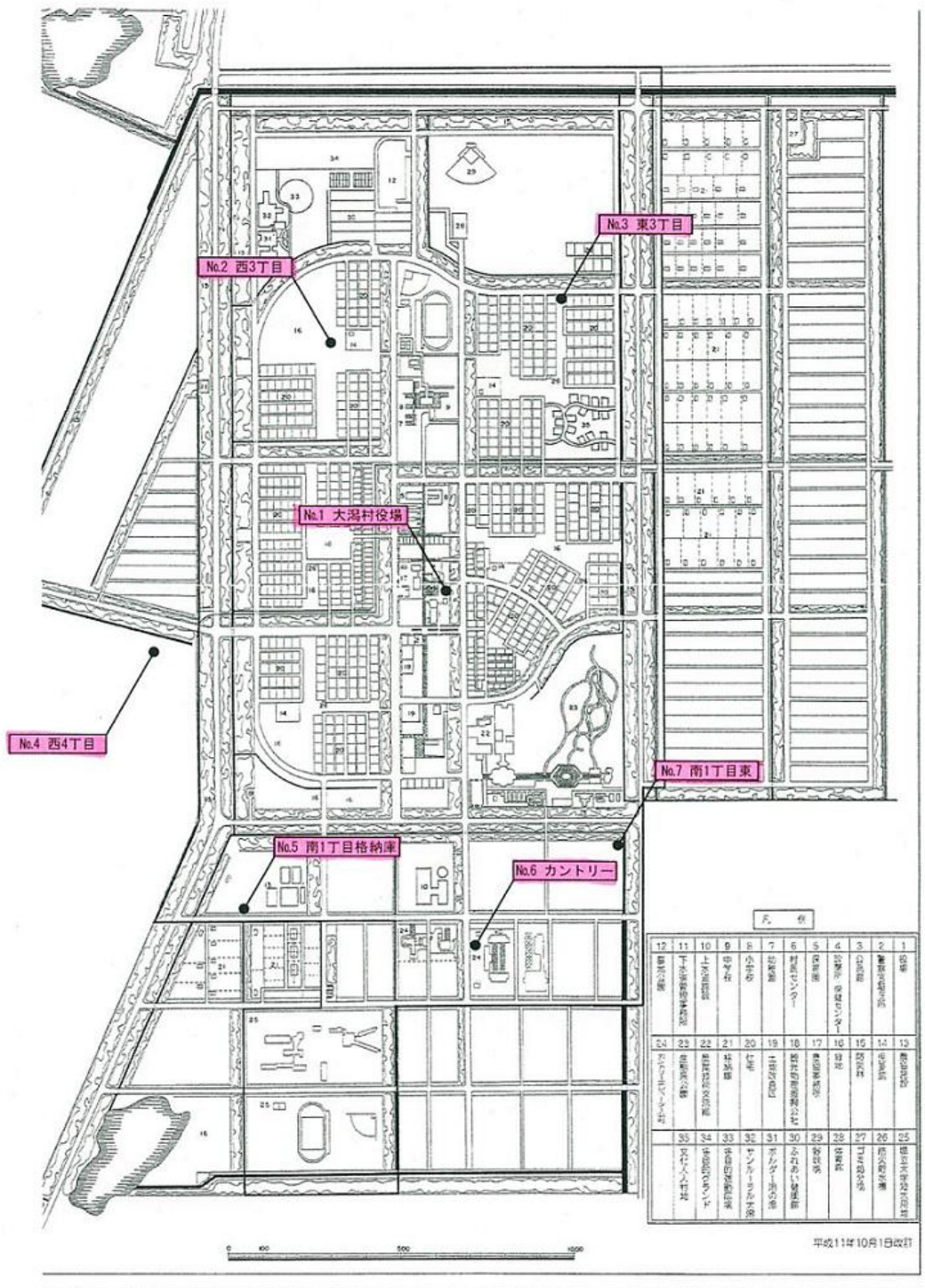
拡声子局配置図
