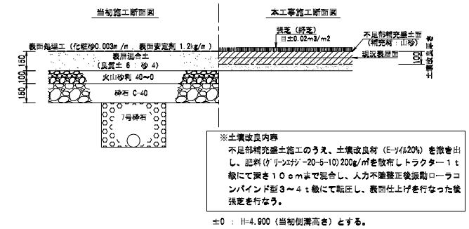
芝生化改良土グラウンド舗装標準断面図 S=1:20
