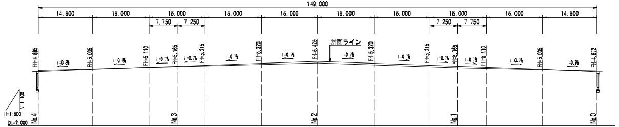
縦断面図
