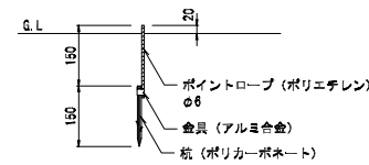
ポイントマーク 詳細図 S=1:10
