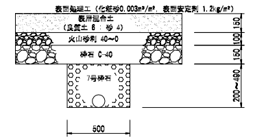
クレイ舗装標準断面図 S-1/20 ※平成10年12月竣工時
