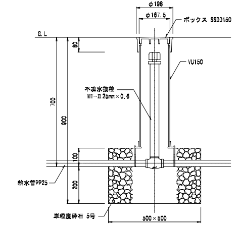
水抜栓 断面図 S-1:10
