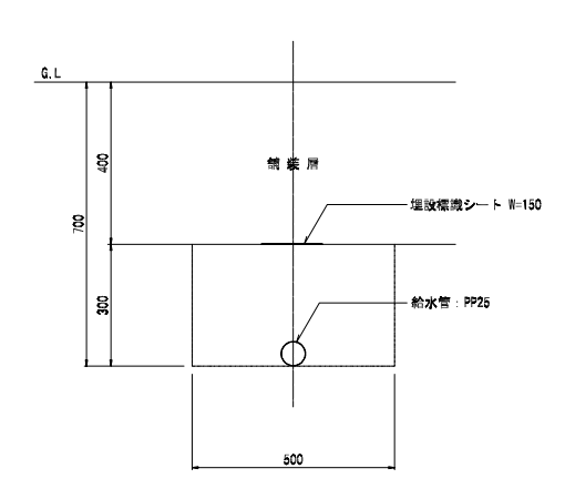
給水管 断面図 S-1:10
