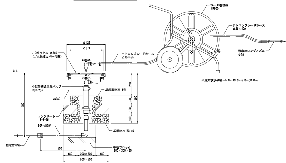
散水栓・散水機器 詳細図 S=1:10
