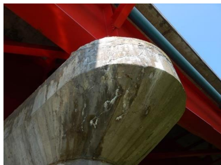
橋脚の遊離石灰を伴うひびわれ
