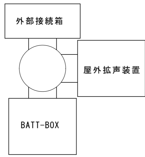
機器装柱図
