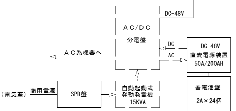
構成図（親局：大潟村役場）
