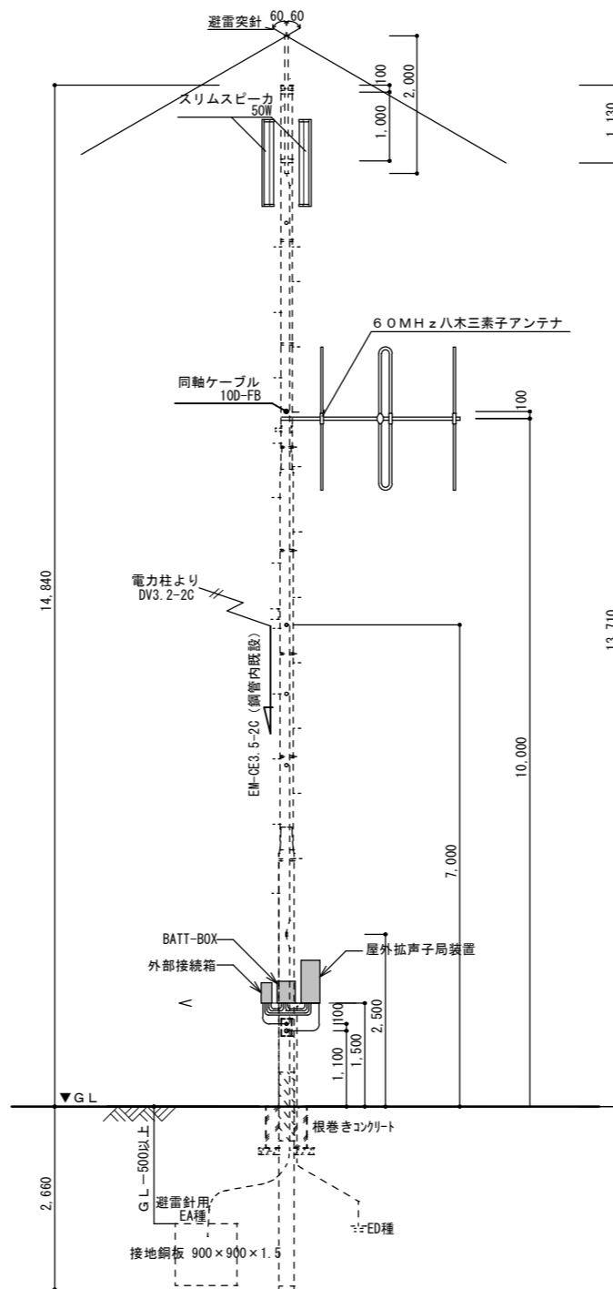
新設屋外拡声子局装柱図 1 : 100
