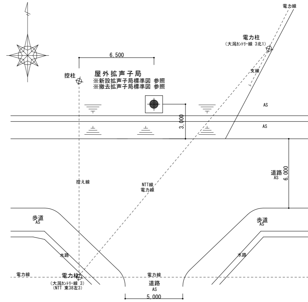
配置図 1:200
