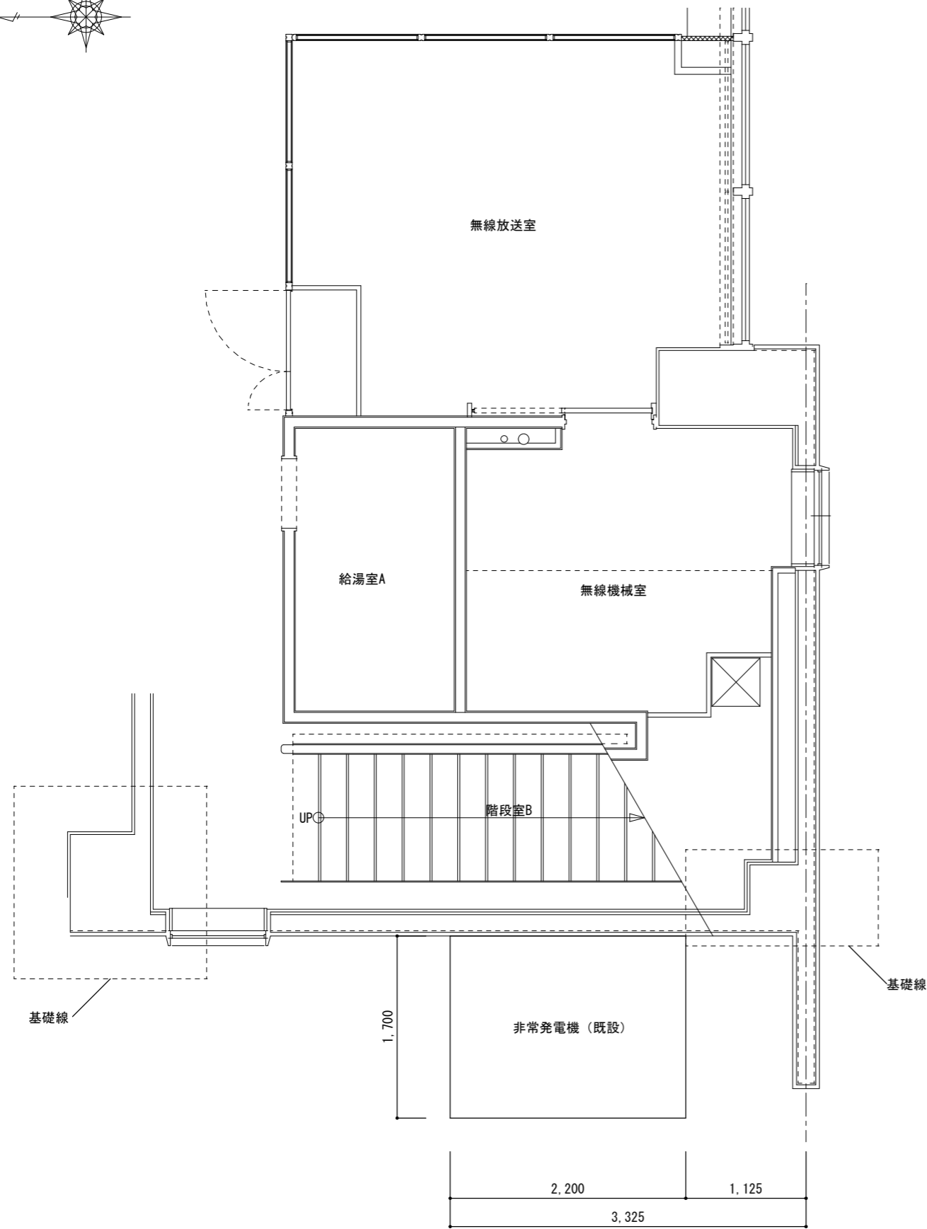
外部機器配置図
