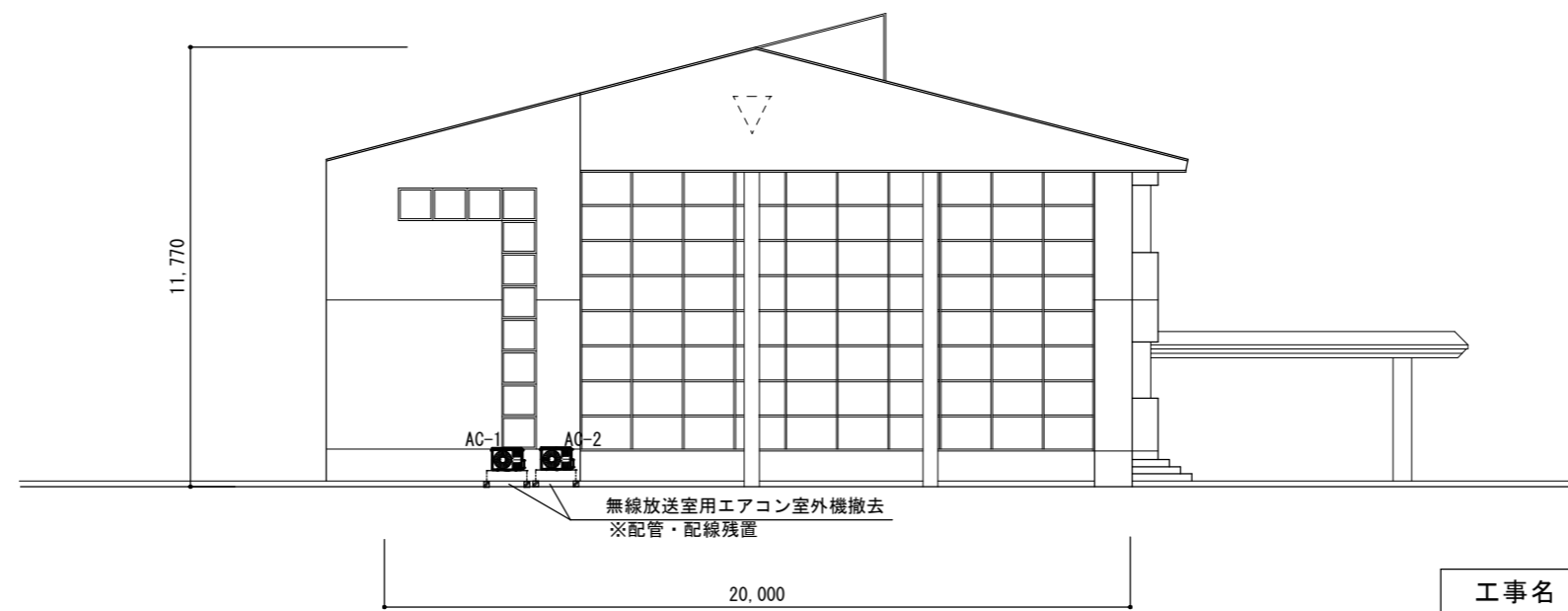
南立面図 1 : 200
