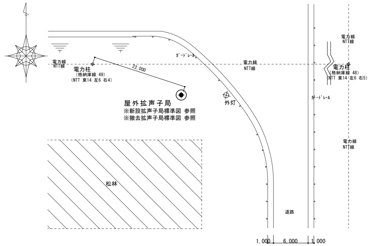
配置図 1 : 400
