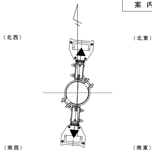
スピーカ方向図
