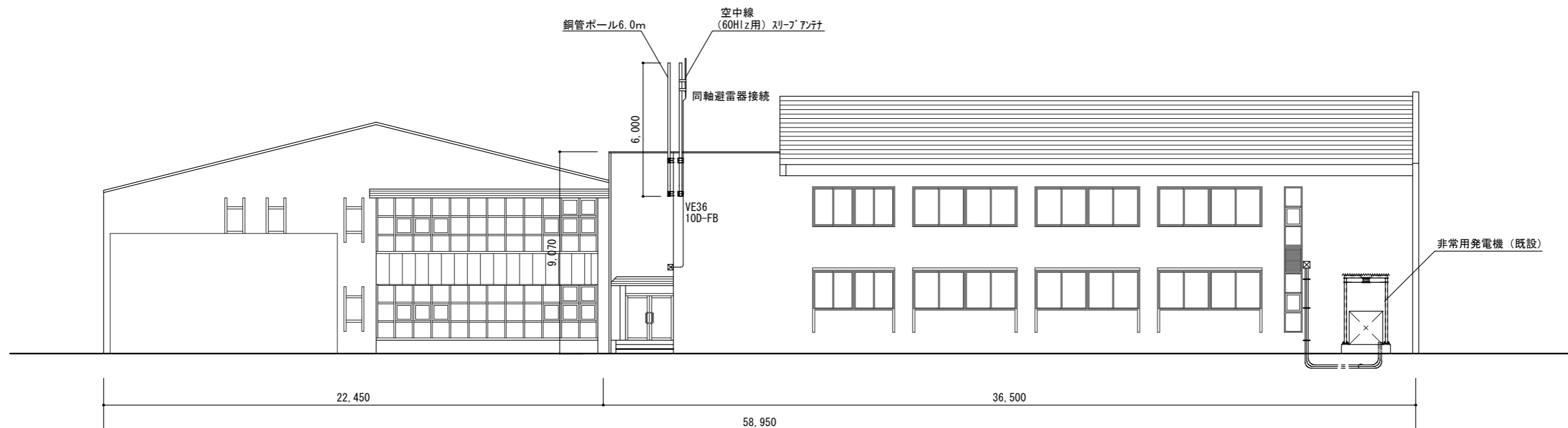
西立面図 1 : 200
