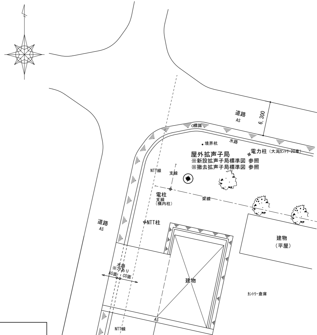
配置図 1:400
