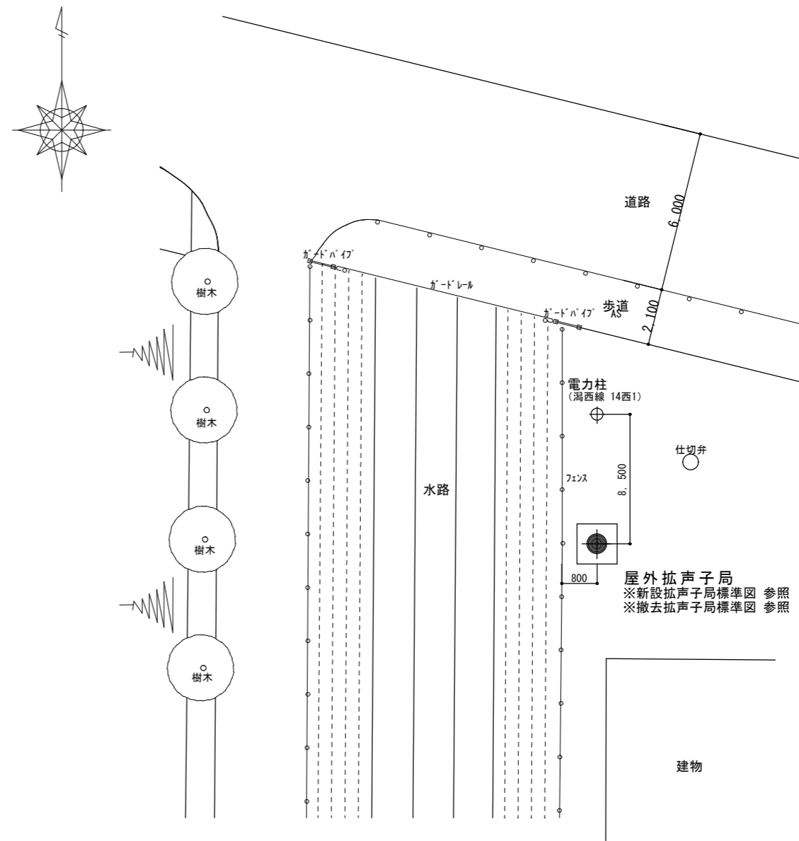
配置図 1:200
