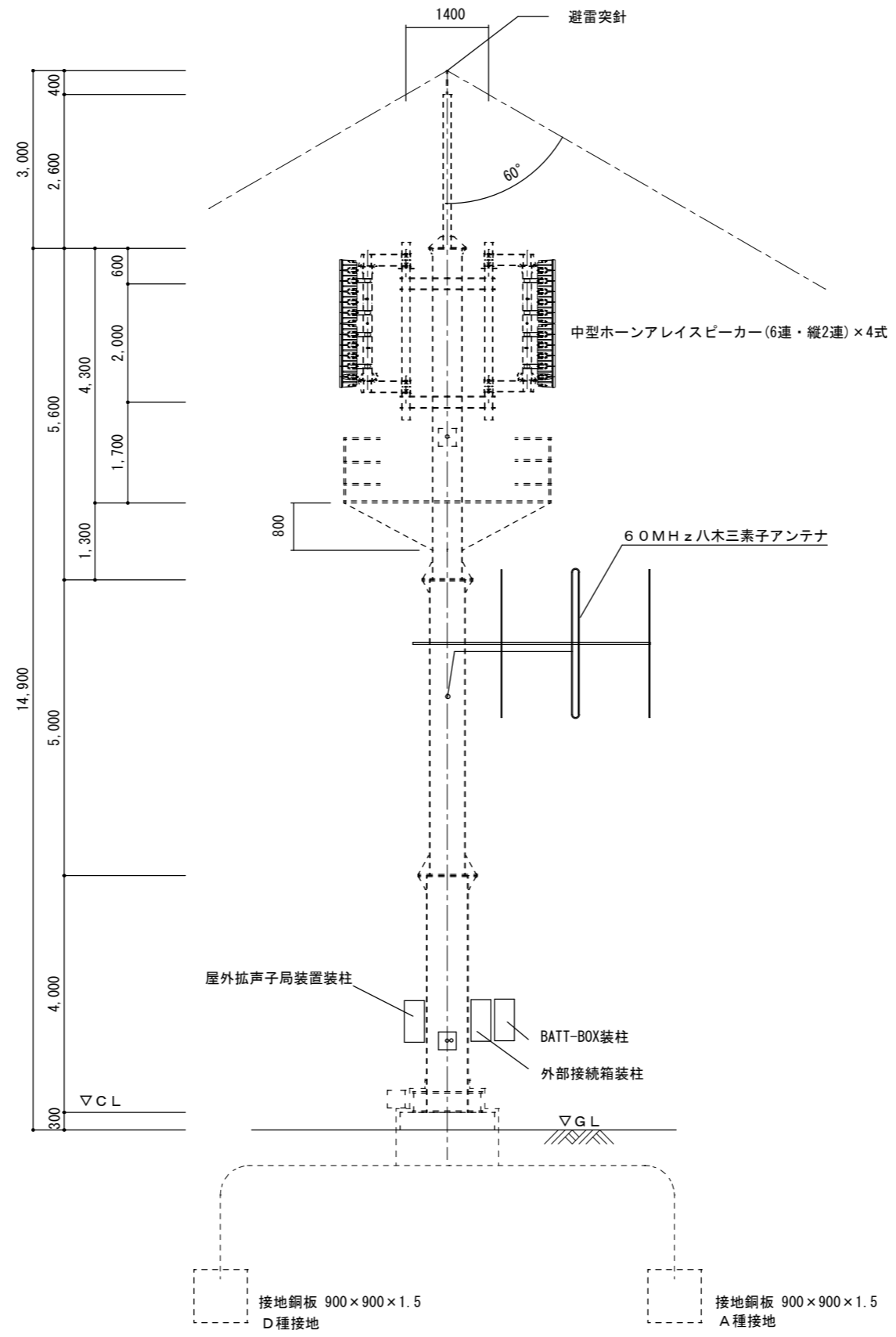
鉄塔姿図 1:100
