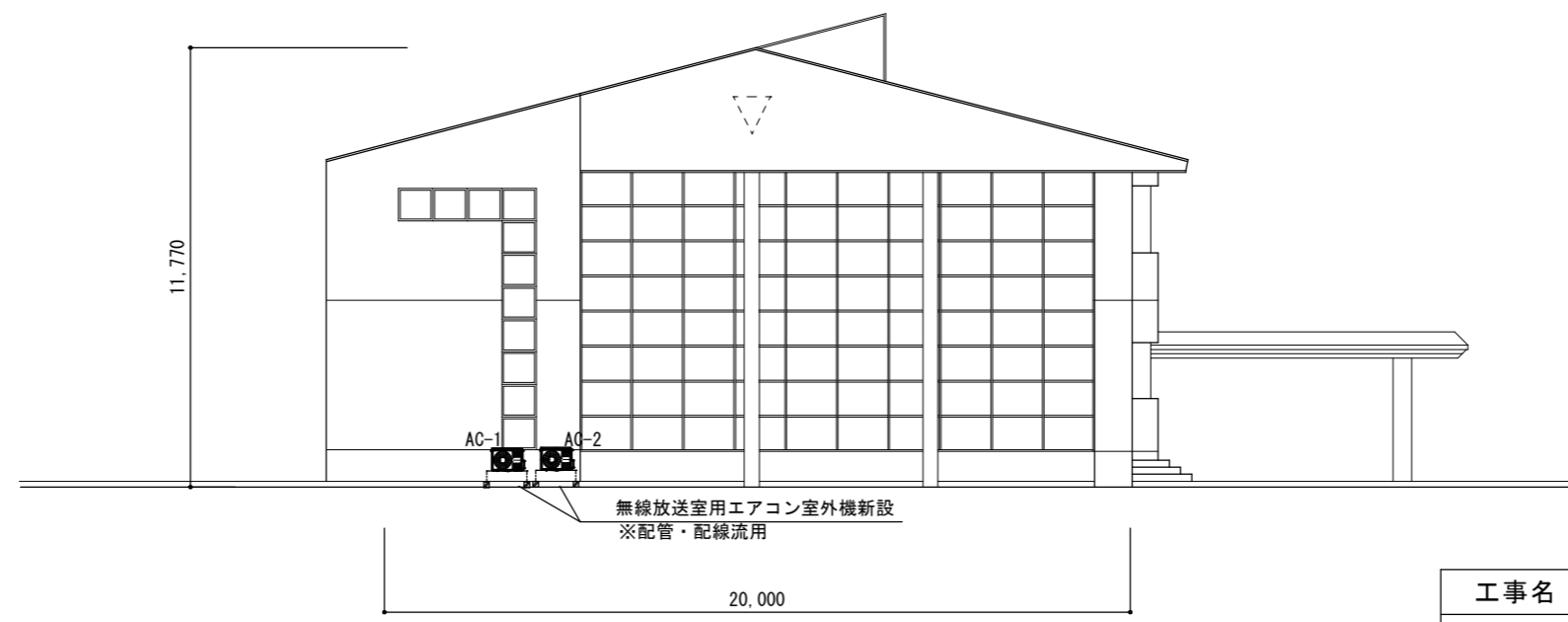
南立面図 1 : 200
