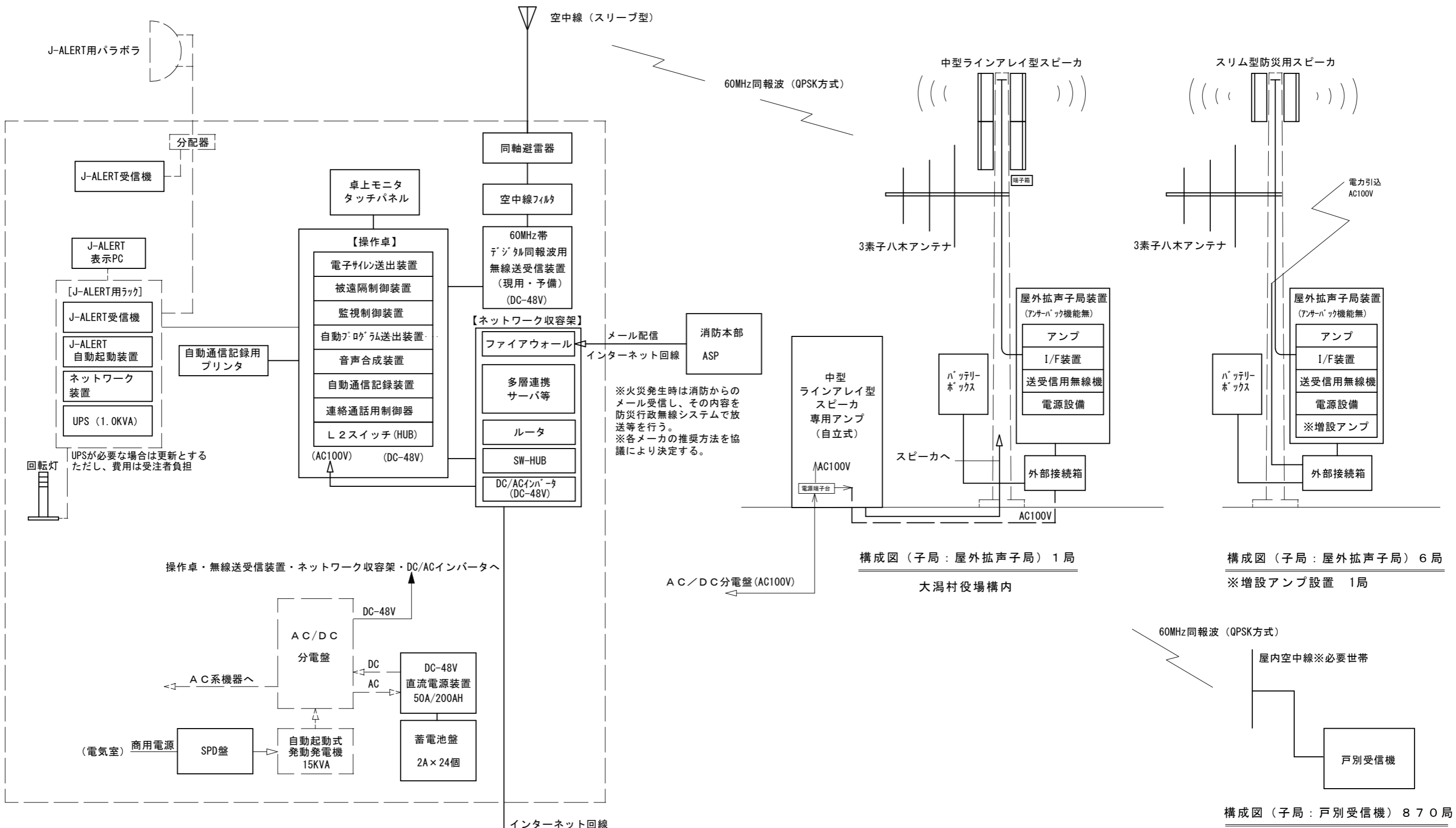
構成図（親局：大潟村役場）
