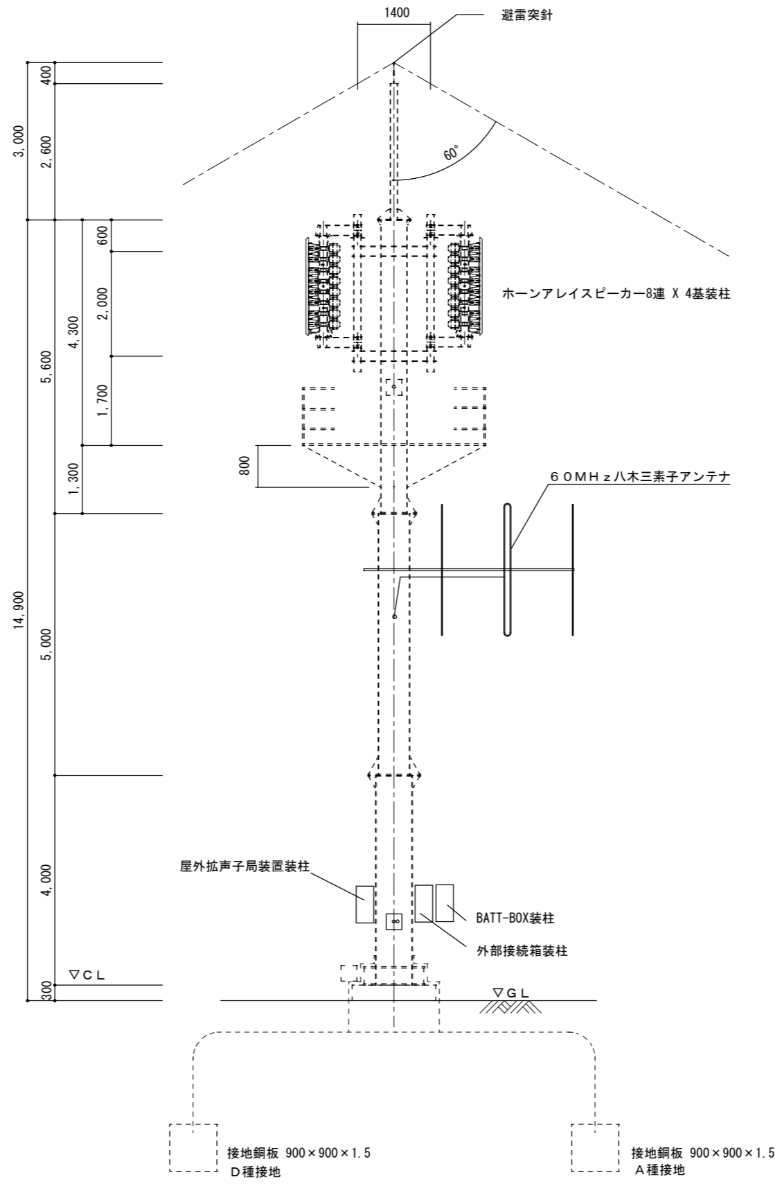
鉄塔姿図 1:100
