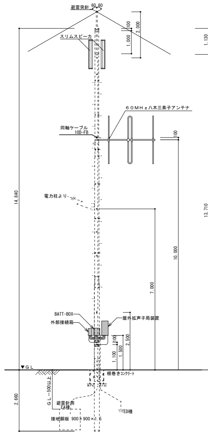
撤去屋外拡声子局装柱図 1 : 100
