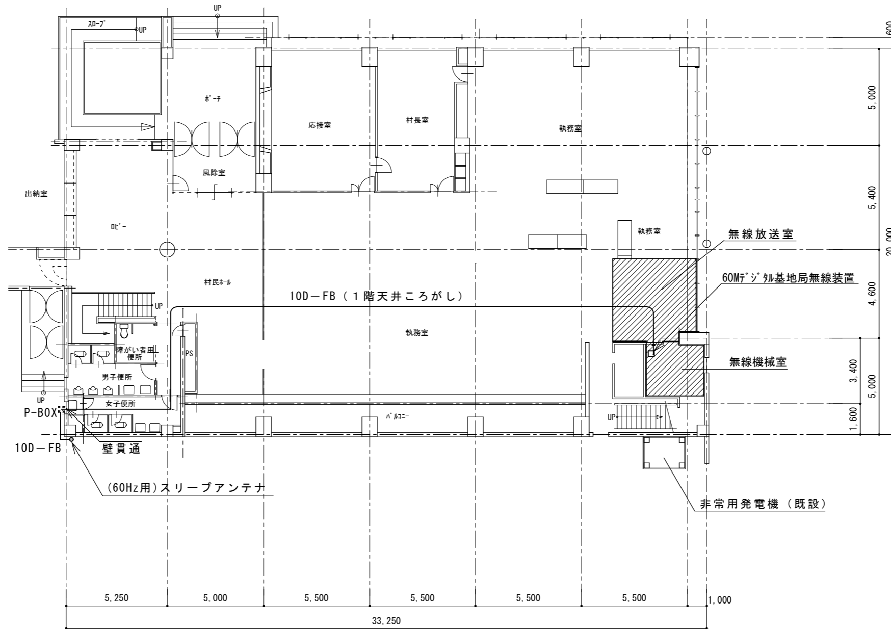
1階平面図 1:200
