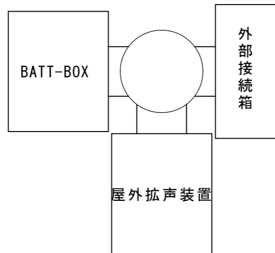
機器装柱図
